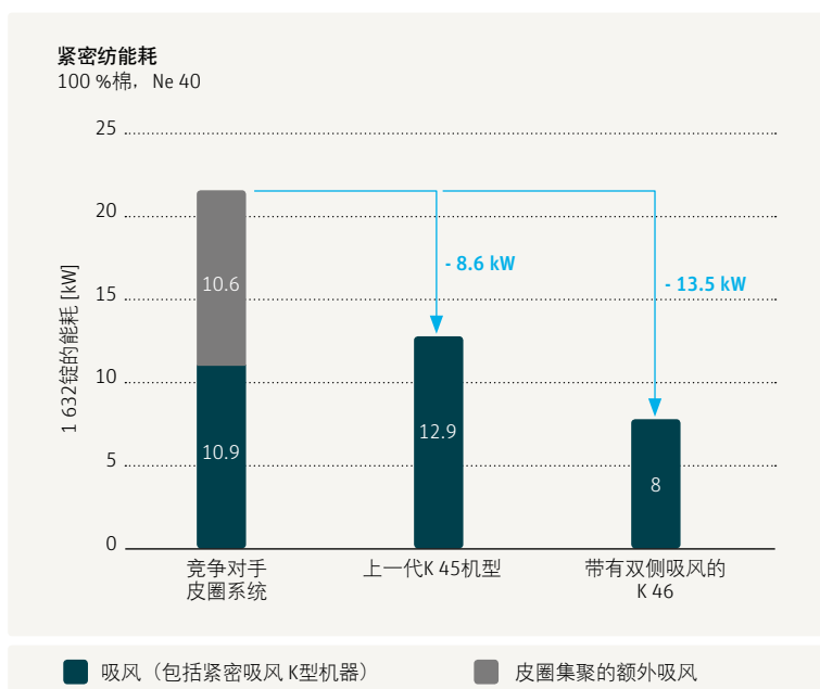
图3 紧密纺纱机K 46与其他传统环锭细纱机相比，所需能耗更低。
